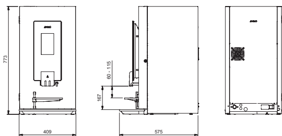
ZIJAAZICHT RECHTS
