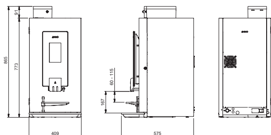
ZIJAAZICHT RECHTS
